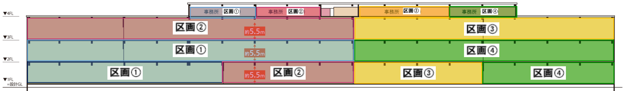
北側断面図
